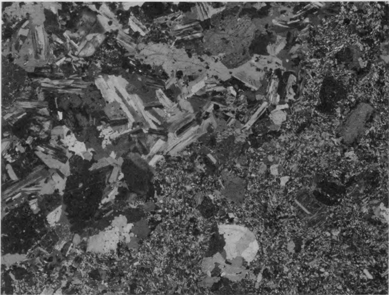
一戸深成岩体の2種類のモンゾニ岩の関係を示す薄片写真(写真の横幅は22mm)
